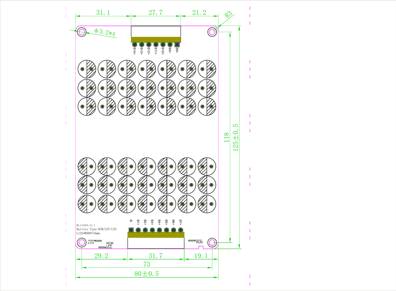
Габаритный чертеж EK-C14S5A. Размеры указаны в миллиметрах.
