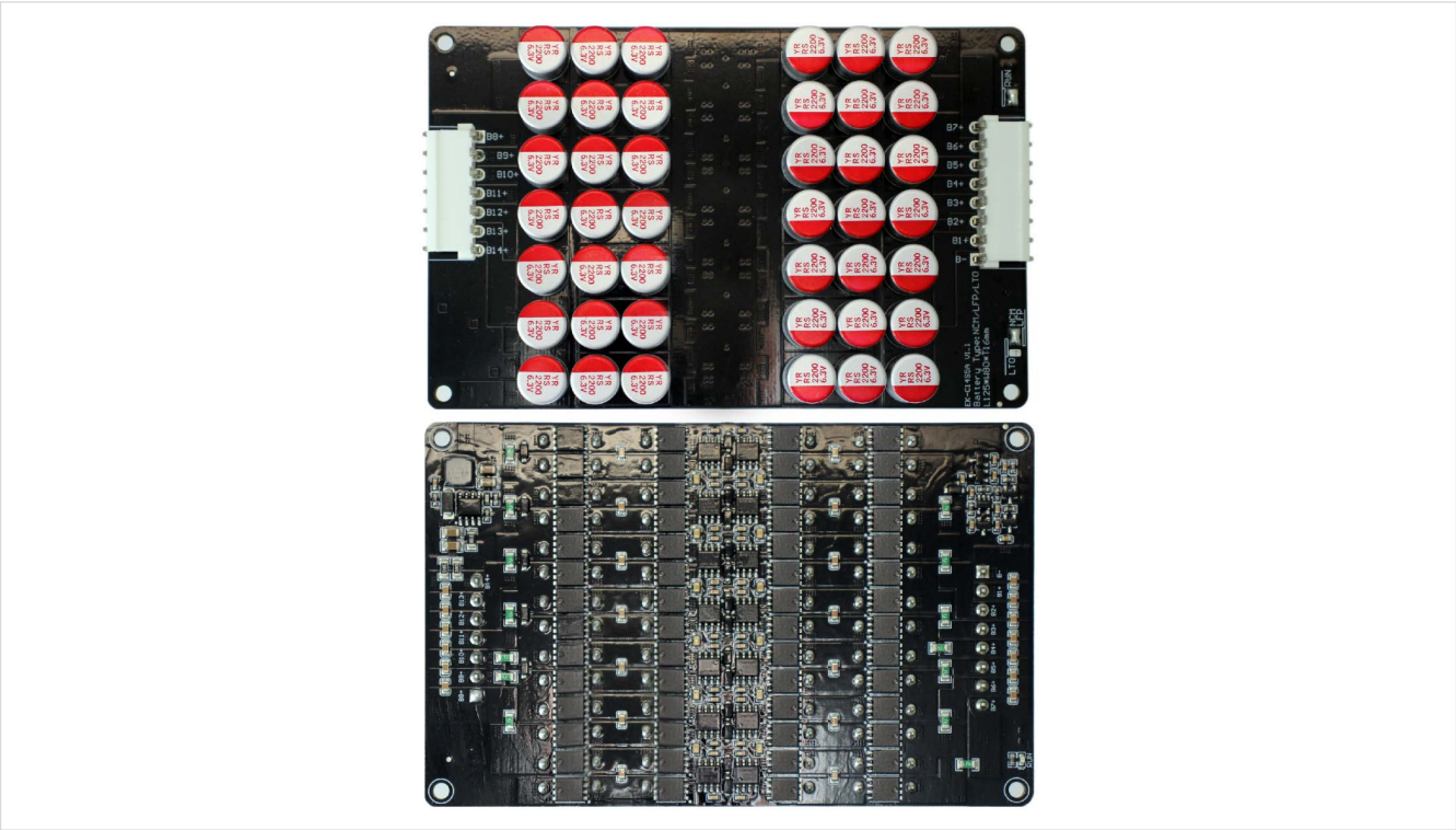
Плата EK-C14S5A с конформным защитным покрытием.
